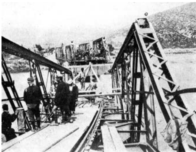
Εικ. 10. Γέφυρα στο Σιδηρόκαστρο, την οποία κατέστρεψαν οι υποχωρούντες Βούλγαροι.
